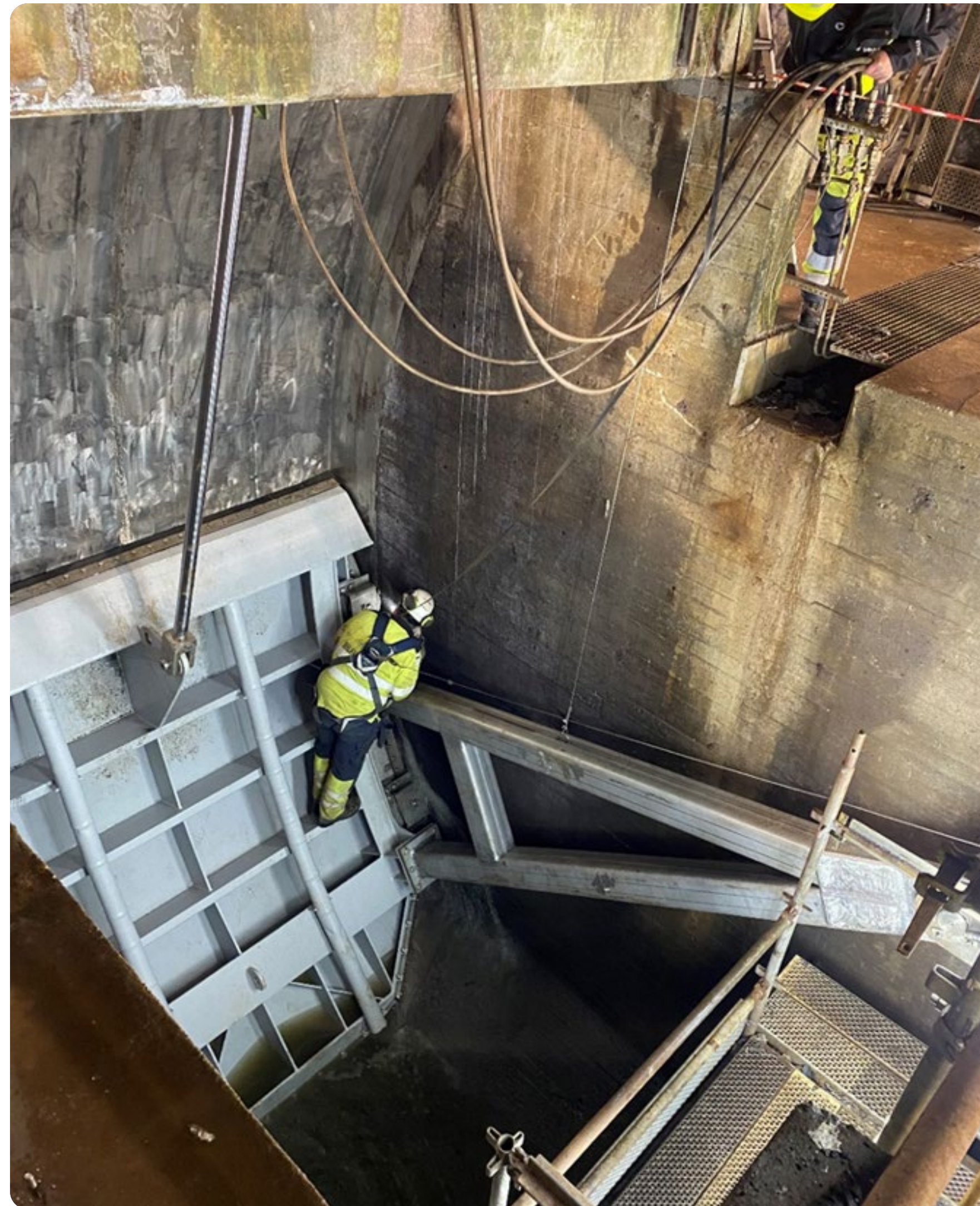
Den store reguleringsluken ved Engervann i Bærum ble rehabilitert i 2023.
