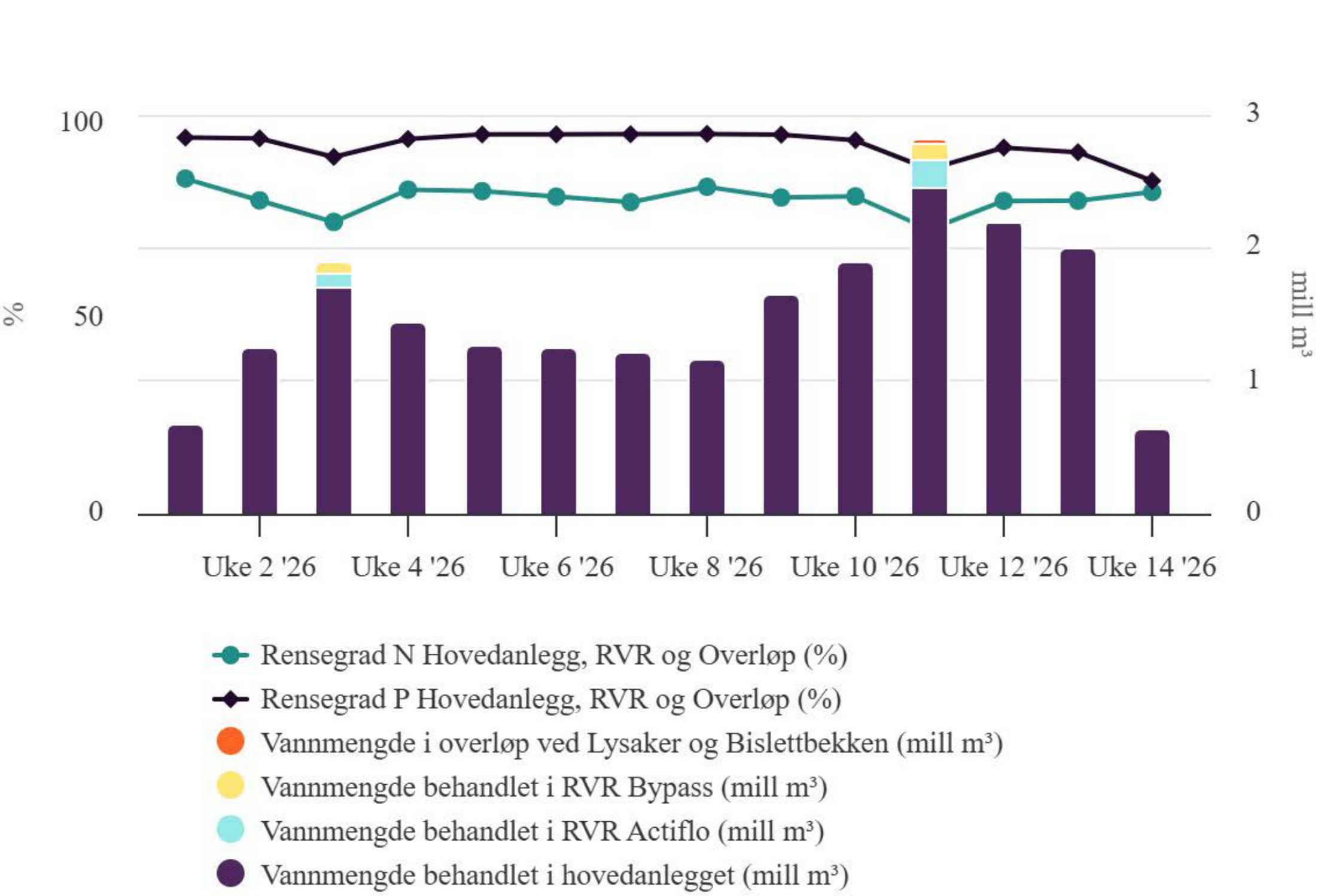
Behandlet vannmengde, nitrogen- og fosforrensegrad Veas 2026 29.12.2025 - 31.03.2026
