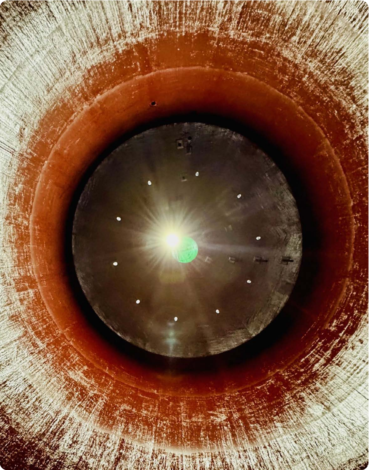
En av Veas' utråtningsstanker sett fra innsiden.
